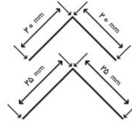
پروفیل L
