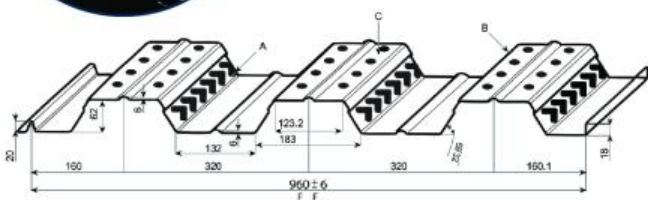
عرشه فولادی (گام ۶۵ و ۷۵)
